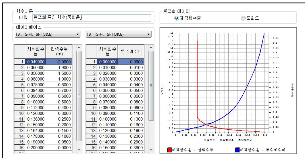
【그림 20.15】 압력수두-체적함수물(포화도)-투수계수비 함수
